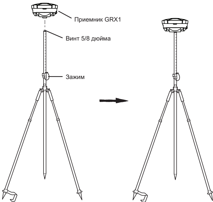
Рис. 4-2. Крепление GRX1 на вешке к биподу
