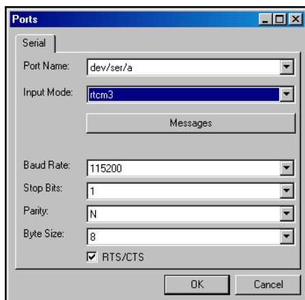
Рис. 3-17. Настройка портов
