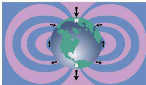
Рис. 9. Дипольное электромагнитное поле Земли.
