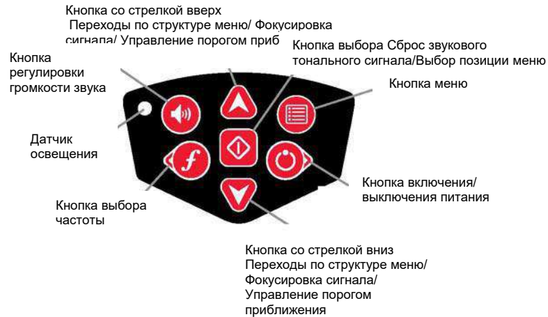
Рис. 5. Кнопочный пульт.
