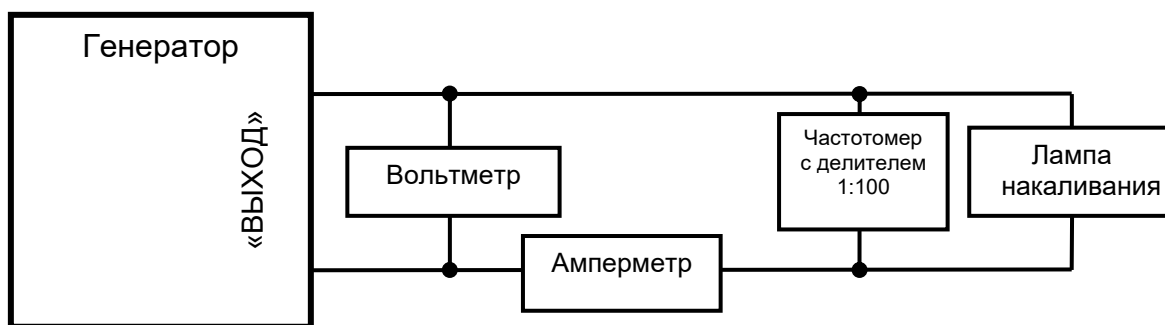
Рисунок 7.5.3 – Схема рабочего места для проверки параметров генератора
