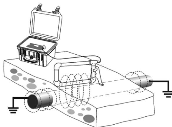
б) ГТ-75
