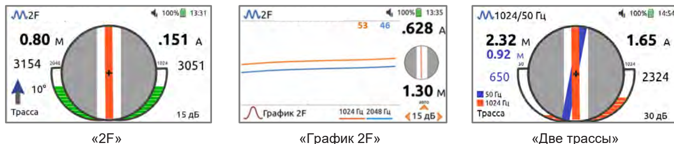
Рисунок 3.2. Виды индикации в двухчастотных режимах.
