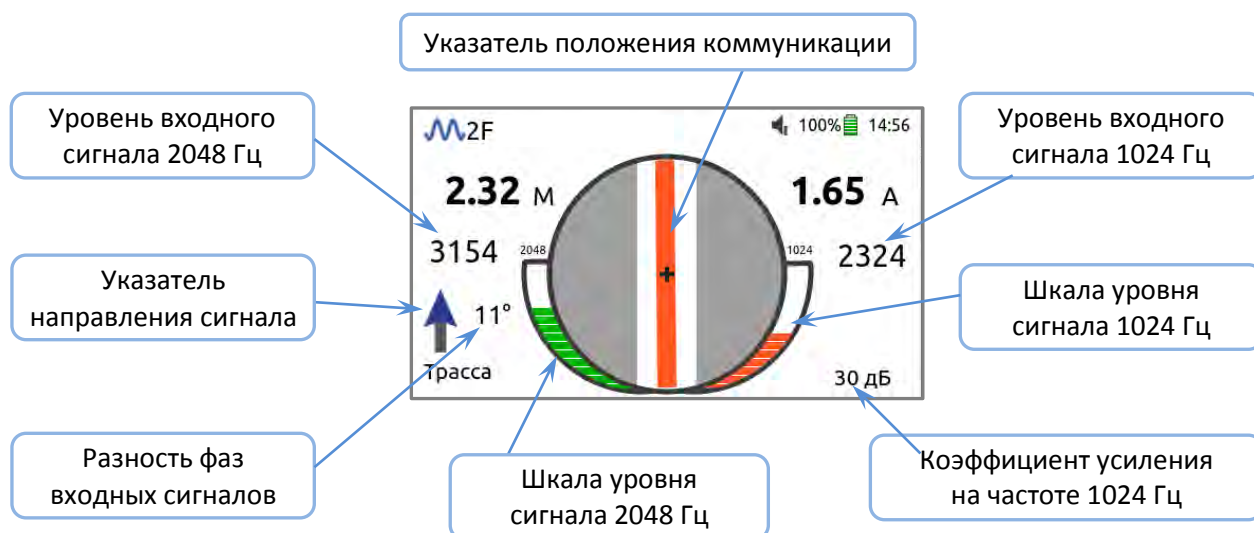
Рисунок 3.15. Режим «Трасса» при двухчастотном режиме.
