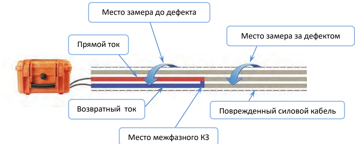
Рисунок Б.4. Определение места межфазного КЗ методом возвратного тока.
