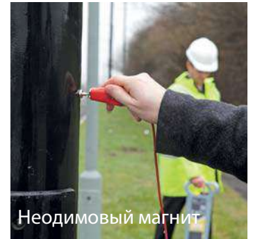
Способ трассировки кабелей малого диаметра
