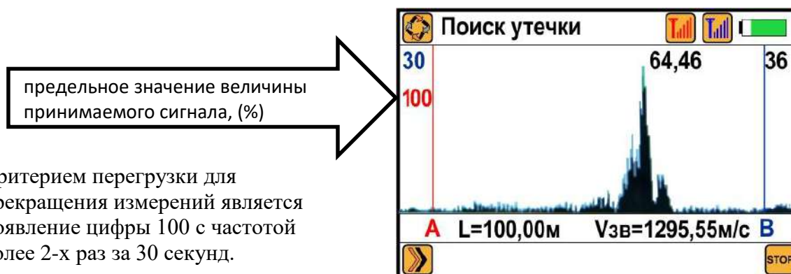
Рисунок 7 Перегрузка принимаемого сигнала
