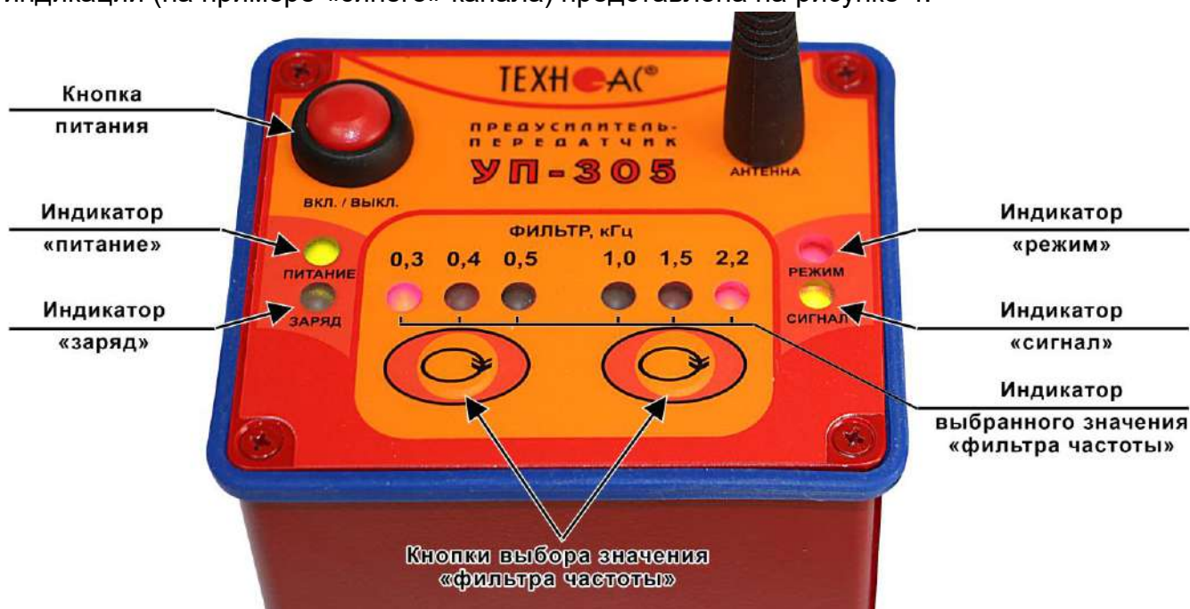
Рисунок 4 Органы управления и индикации «УП-305»
