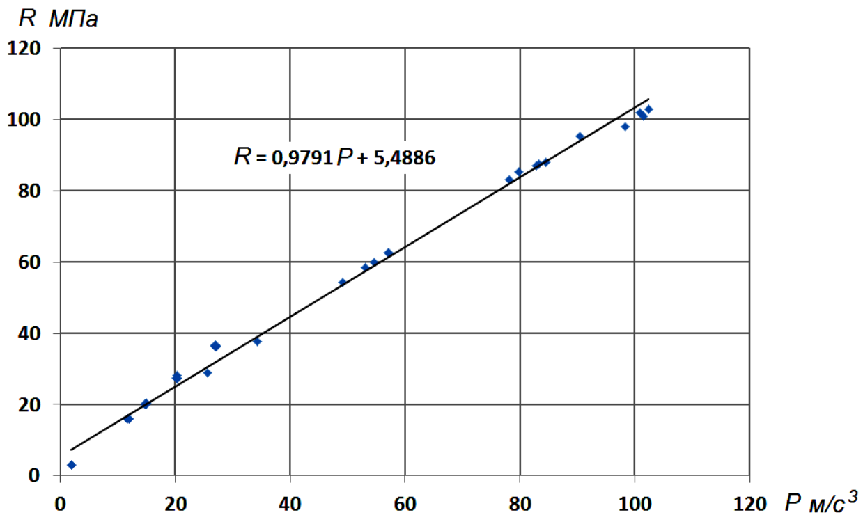
Рисунок 1 – Построение линейной градуировочной зависимости между параметром Р и прочностью бетона R
