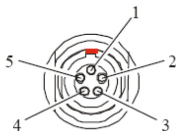
Разъем Данные / Питание PDL 450
