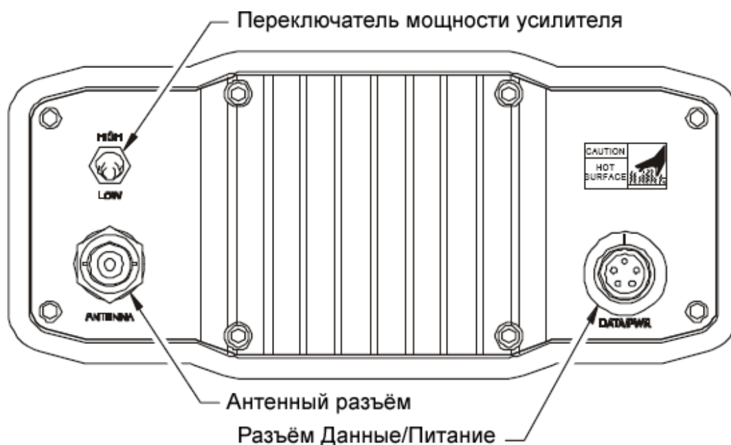
Рисунок 5 - Задняя панель HPB 450
