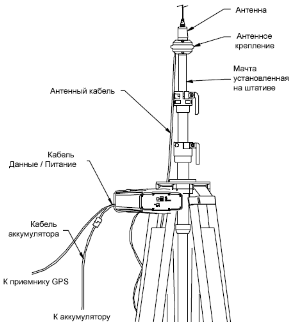
Рисунок 6 - Установка HPB 450
