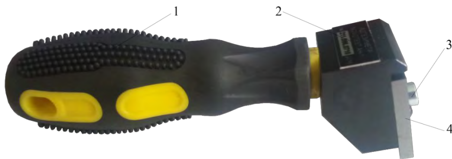
1 – ручка; 2 – информация о приборе; 3 – болт; 4 – резак.
